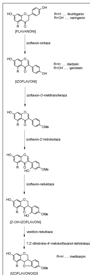
Slika 4: Pretvorba flavanonov (1, 8).
