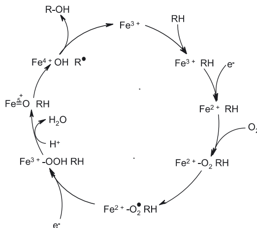
Slika 2: Predpostavljen katalitski mehanizem oksidacije s citokromom P450. RH = substrat (2)
