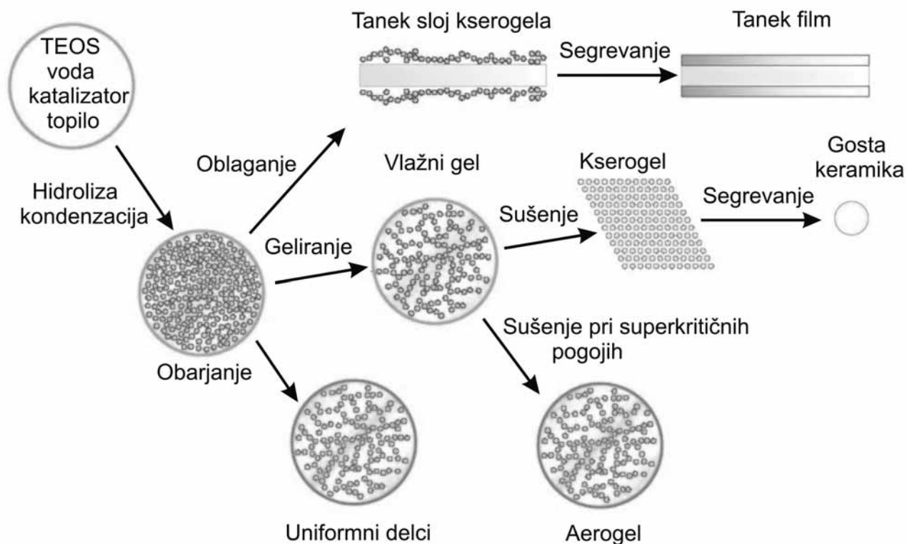
Slika 1: Pregled sol-gel postopka z nekaterimi aplikacijami (9).
