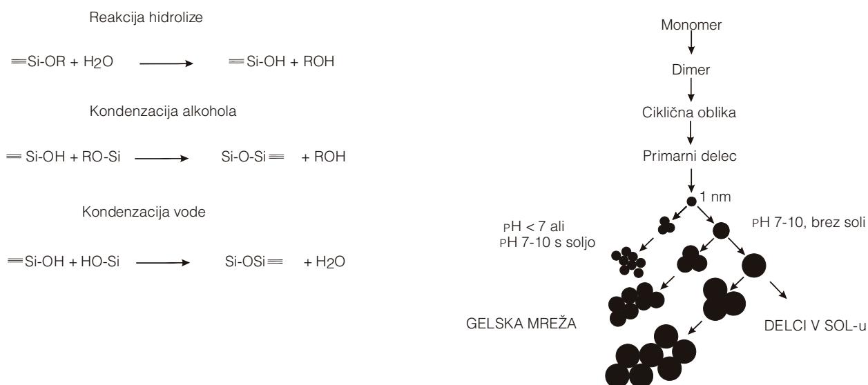
Slika 2: Reakcije alkoksilanov (10) in tvorba silicijevega dioksida iz sol-gel postopka s TEOS (11).
