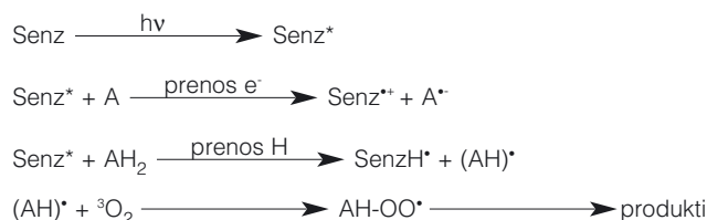
Shema 1. Nastajanje reaktivnih kisikovih intermediatov po zajetju fotona na molekuli fotosenzibilizatorja (Senz). \text{Senz}^* je vzbujeno stanje senzibilizatorja, \text{Senz}^{*+} je kationski radikal senzibilizatorja, A^- anionski radikal substrata.
